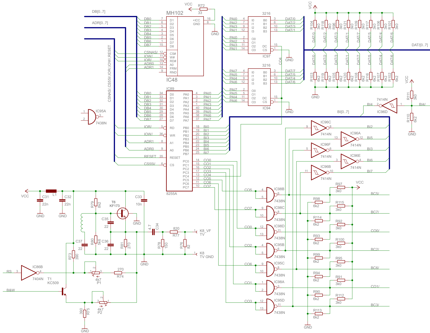
VF MODULATOR, NASOBICKA, PARARELNI MEZISTYK
